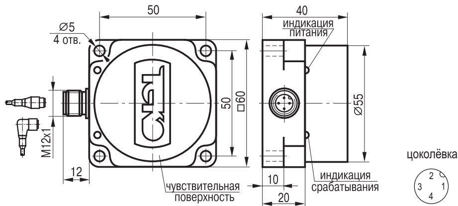
Габаритный чертеж
